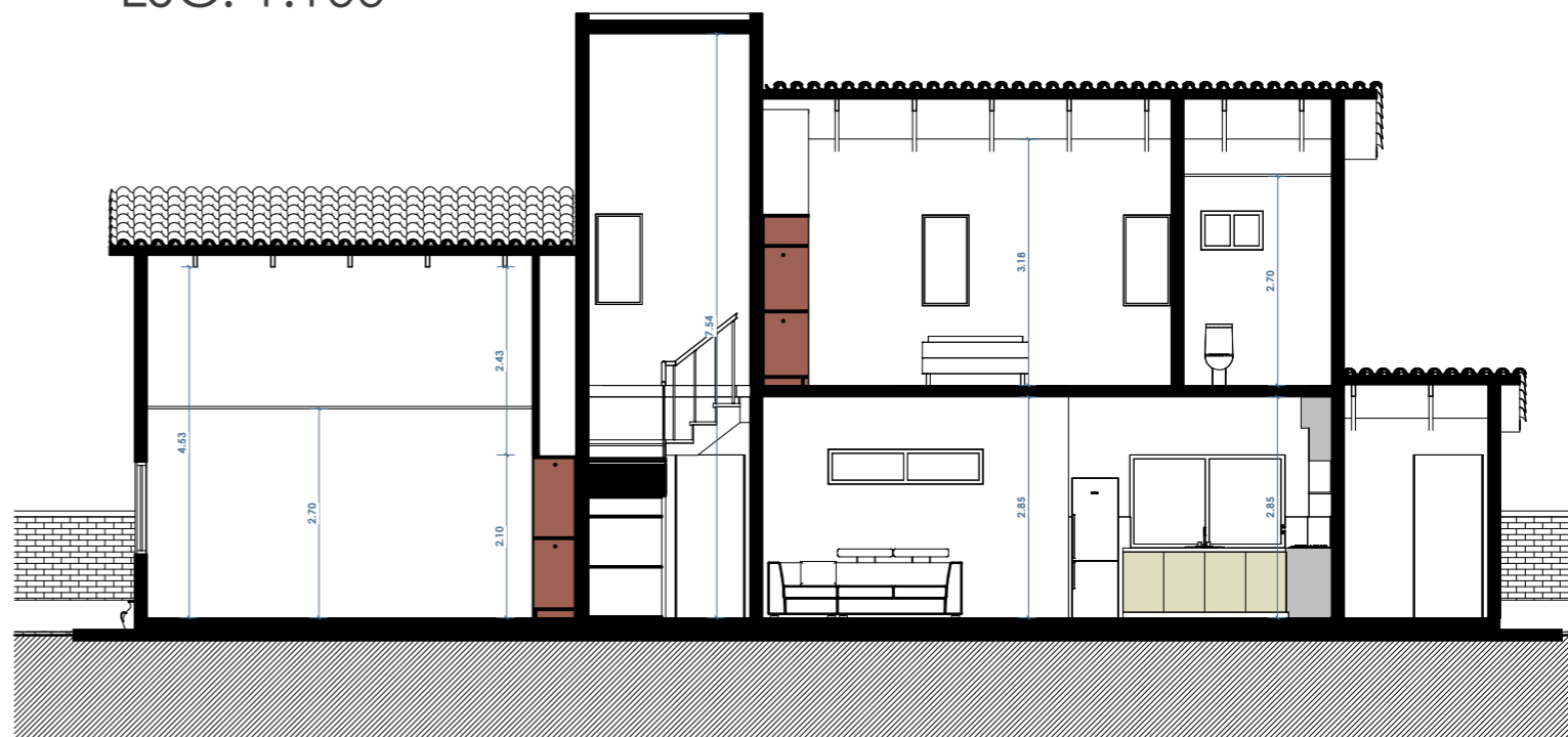
SECCIÓN 4 ESC. 1:100
