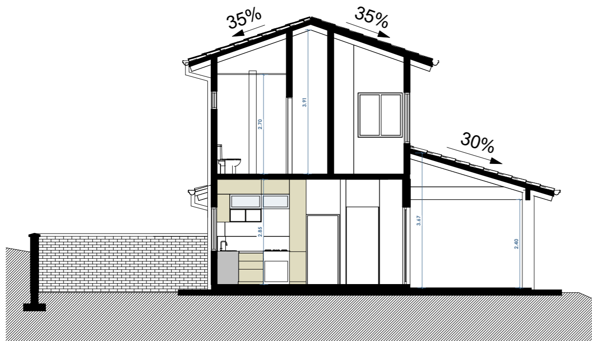
SECCIÓN 3 ESC. 1:100
