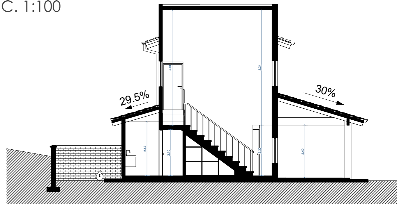
SECCIÓN 4 ESC. 1:100
