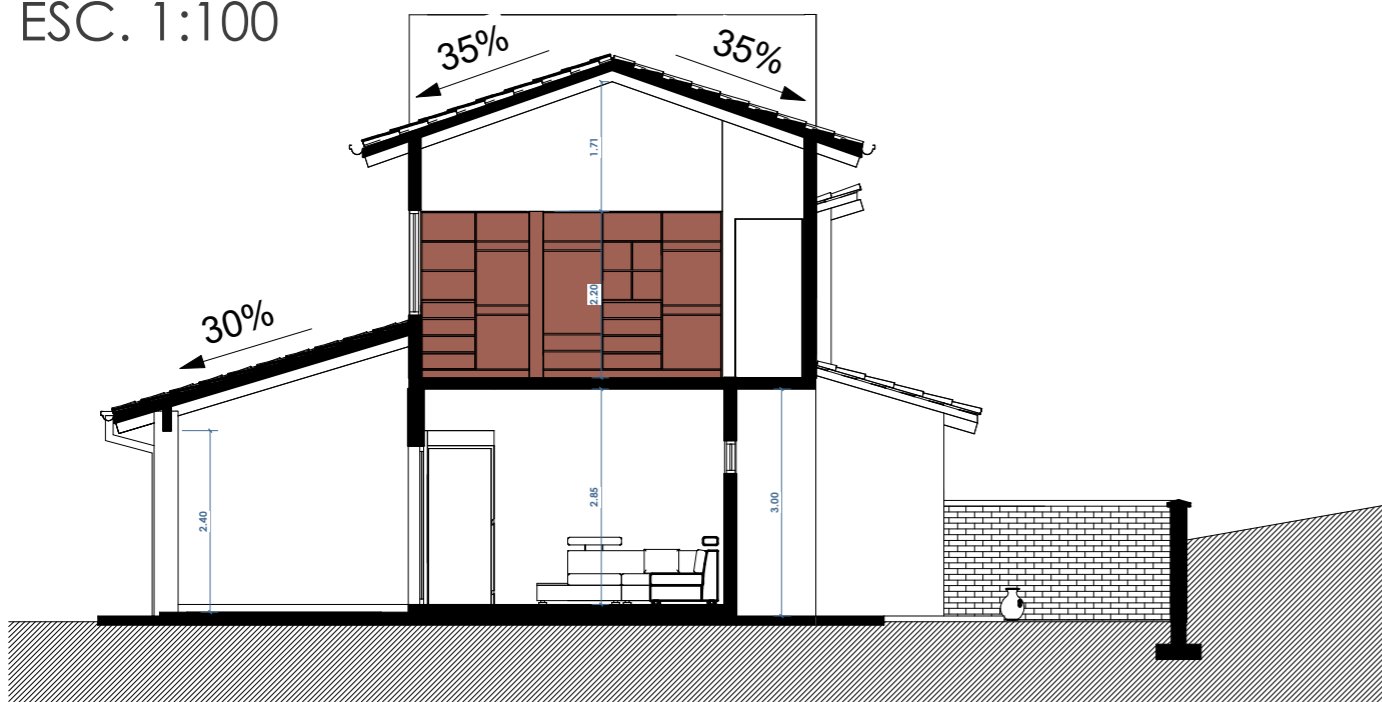
SECCIÓN 3 ESC. 1:100
